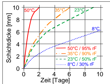
Diagramm 1: Durchhärtungsgeschwindigkeit für Sikasil®-C
