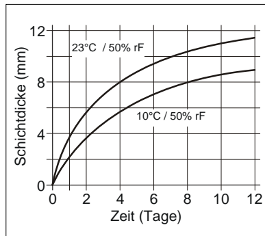
Diagramm 1: Durchhärtungsgeschwindigkeit für Sikaflex®-221
